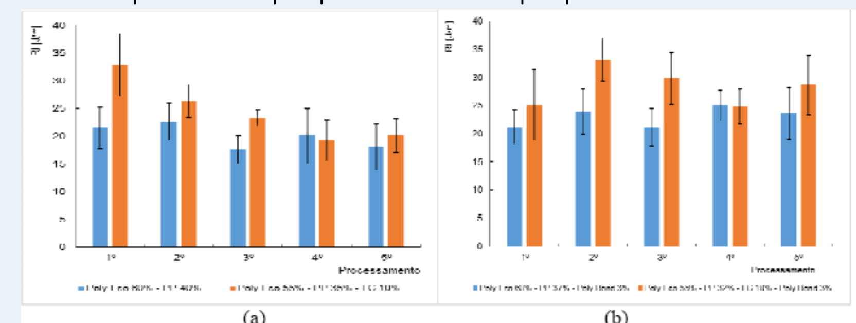
Figura 2: RI dos biocompósitos: (a) PolyEco/PP e PolyEco/PP/FC e (b) PolyEco/PP/PolyBond e PolyEco/PP/FC/PolyBond em função do número de ciclos de reprocessamento.
