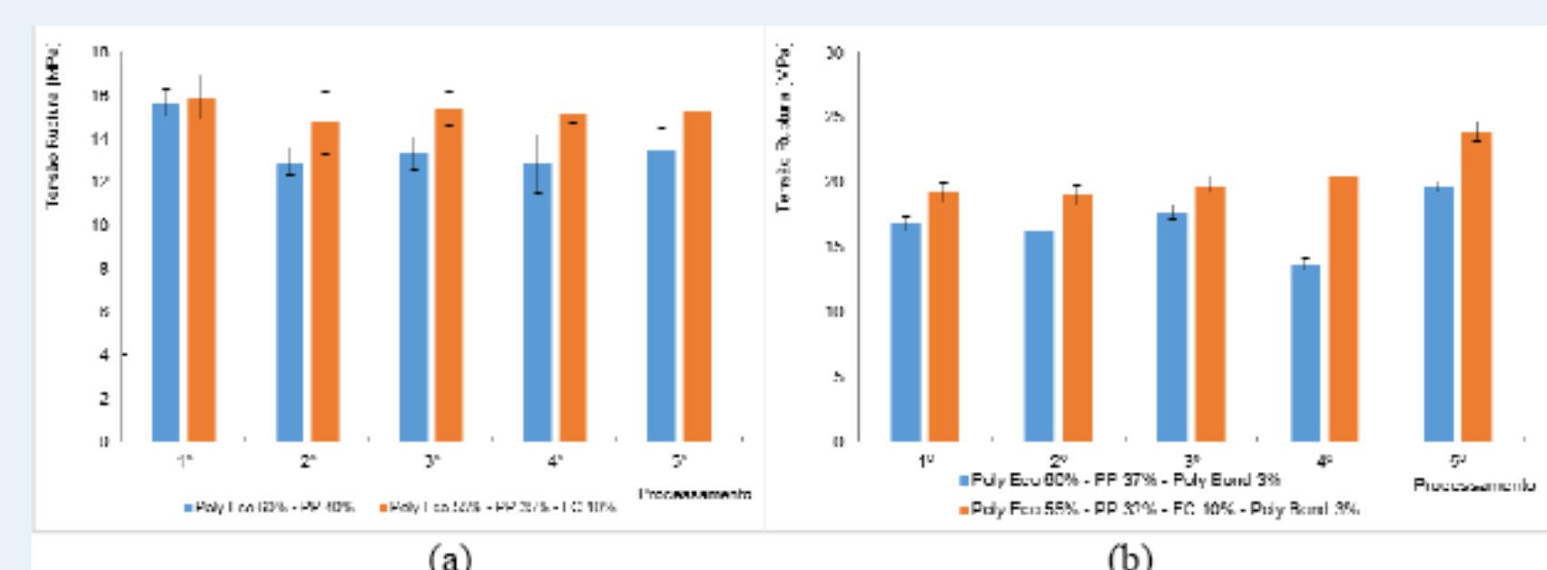
Figura 3: Tensão de Ruptura dos biocompósitos: (a) PolyEco/PP e PolyEco/PP/FC e (b) PolyEco/PP/PolyBond e PolyEco/PP/FC/PolyBond em função do número de ciclos de reprocessamento.
