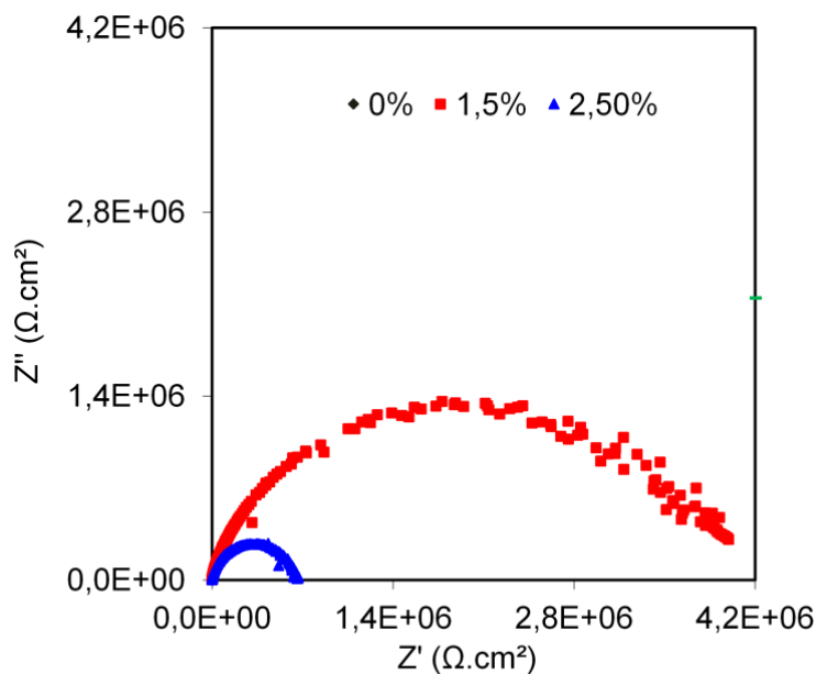
Figura 2: Diagrama de Nyquist no OCP dos revestimentos contendo 0% (◆), 1,5% (■) e 2,5% (▲), após 5 dias de imersão em solução de NaCl 3,5%, pH 2.
