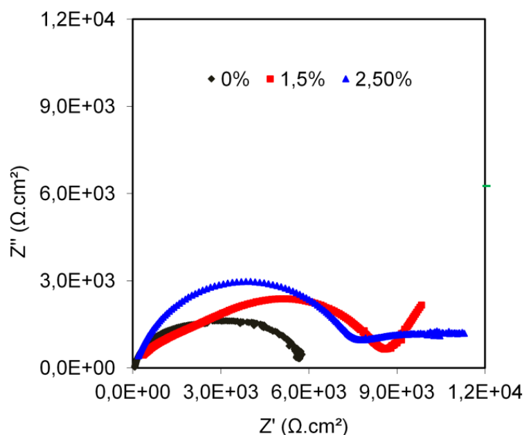
Figura 3: Diagrama de Nyquist no OCP dos revestimentos contendo 0% (◆), 1,5% (■) e 2,5% (▲), após 10 dias de imersão em solução de NaCl 3,5%, pH 2.
