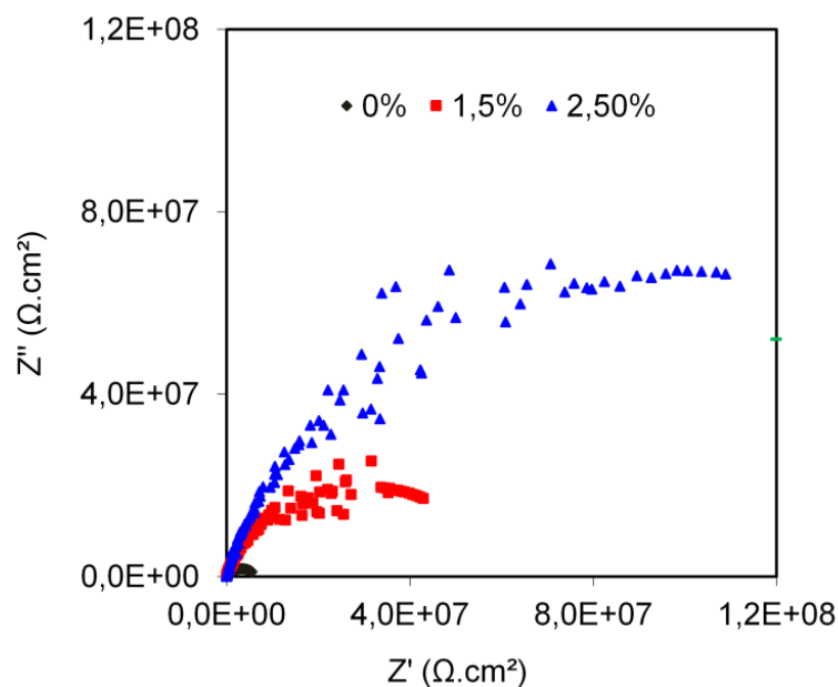
Figura 1: Diagrama de Nyquist no OCP dos revestimentos contendo 0% (♦), 1,5% (■) e 2,5% de ZnO (▲), após 1 h de imersão em solução de NaCl 3,5%, pH 2.
